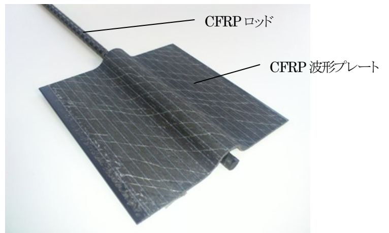
CFRP波形プレート及びCFRPロッド
