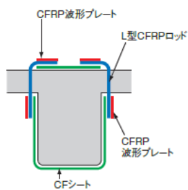
①疑似閉鎖型に巻き付ける場合
