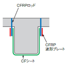
②U字型に巻き付ける場合 (アンカータイプ)
