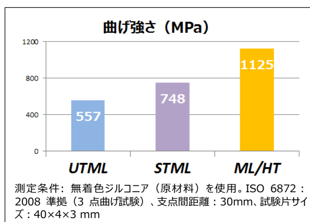
「強度」の比較 (曲げ強さ)
