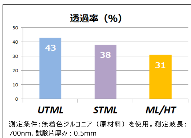
「透光性」の比較 (透過率)
