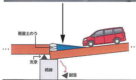
橋梁における段差解消イメージ
