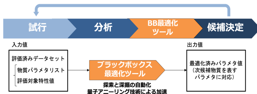
図 1. 量子アニーリングが加速するブラックボックス最適化
