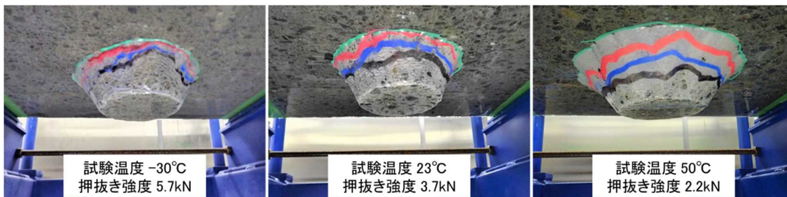
押抜き試験の状況 (50mm 変位時)
