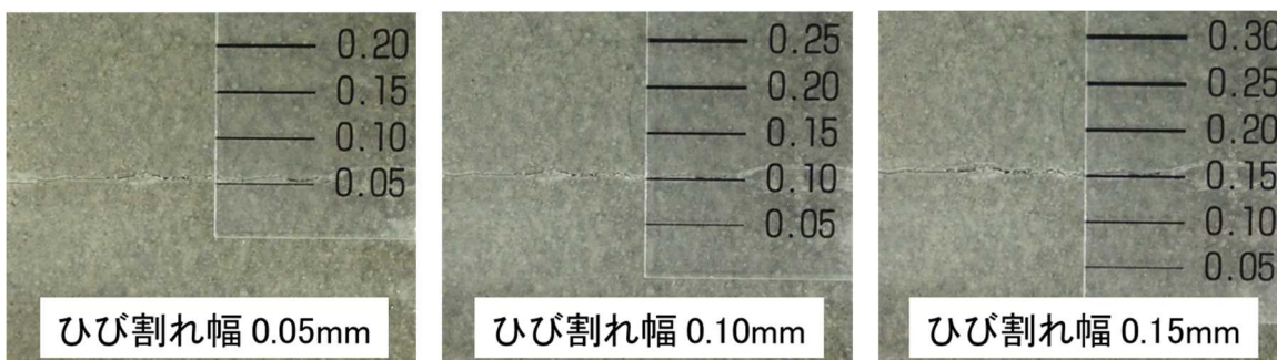
コンクリート下地のひび割れ視認性 (Y 仕様塗布後)
