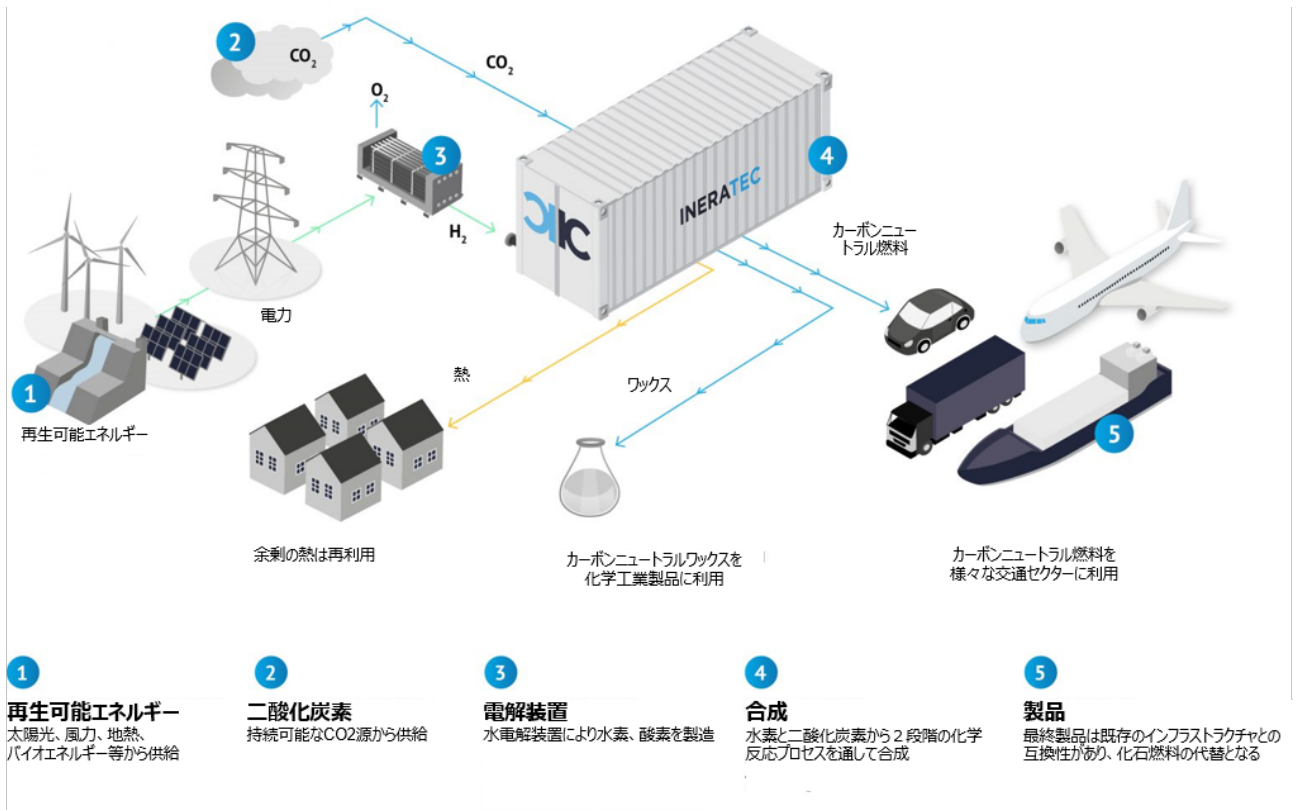
図 1 – 再生可能エネルギーからの e-fuel 製造
