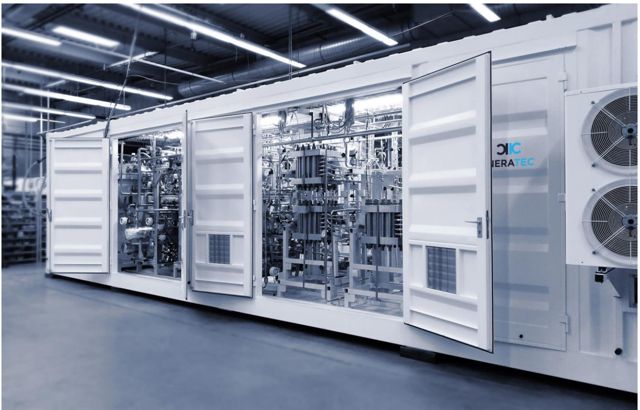
図 2 – INERATEC 社による工業規模のコンテナ型 Power-to-Liquid プラントモジュール(図 1 ステップ④)
