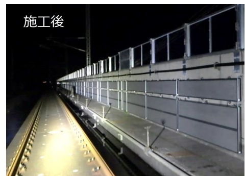
全天候型吸音材を使用した吸音板施工例（上越新幹線 散水区間）
