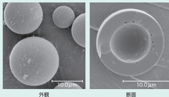
ポリイミド中空微粒子開発品の電子顕微鏡写真
