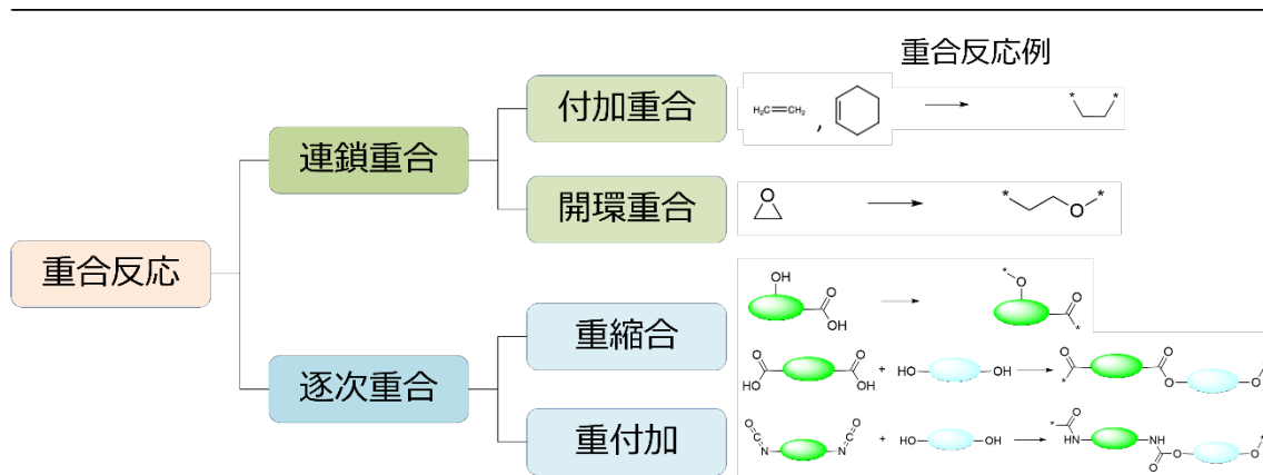
図 1. SMiPoly に実装されている高分子重合反応ルール集合
