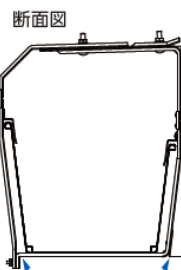
屋根材の伸縮に 追従し易い船底形状
