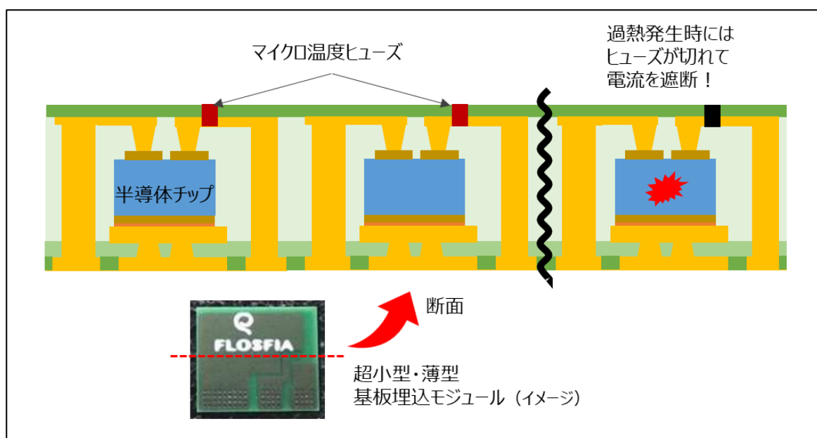
新マイクロ温度ヒューズの動作イメージ
