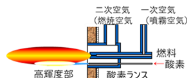
図 1 酸素ランス方式
