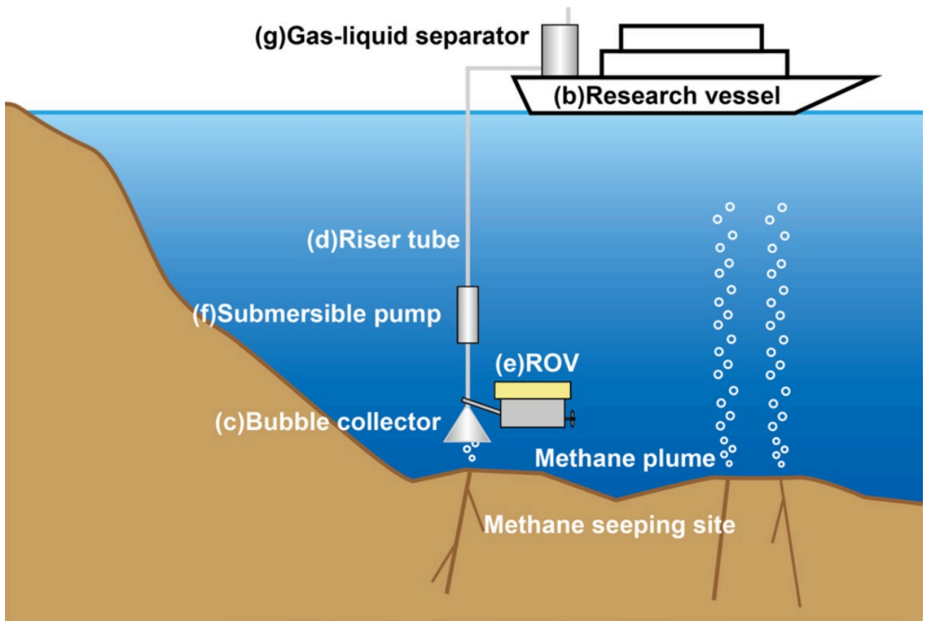
メタンブルーム回収概念図
