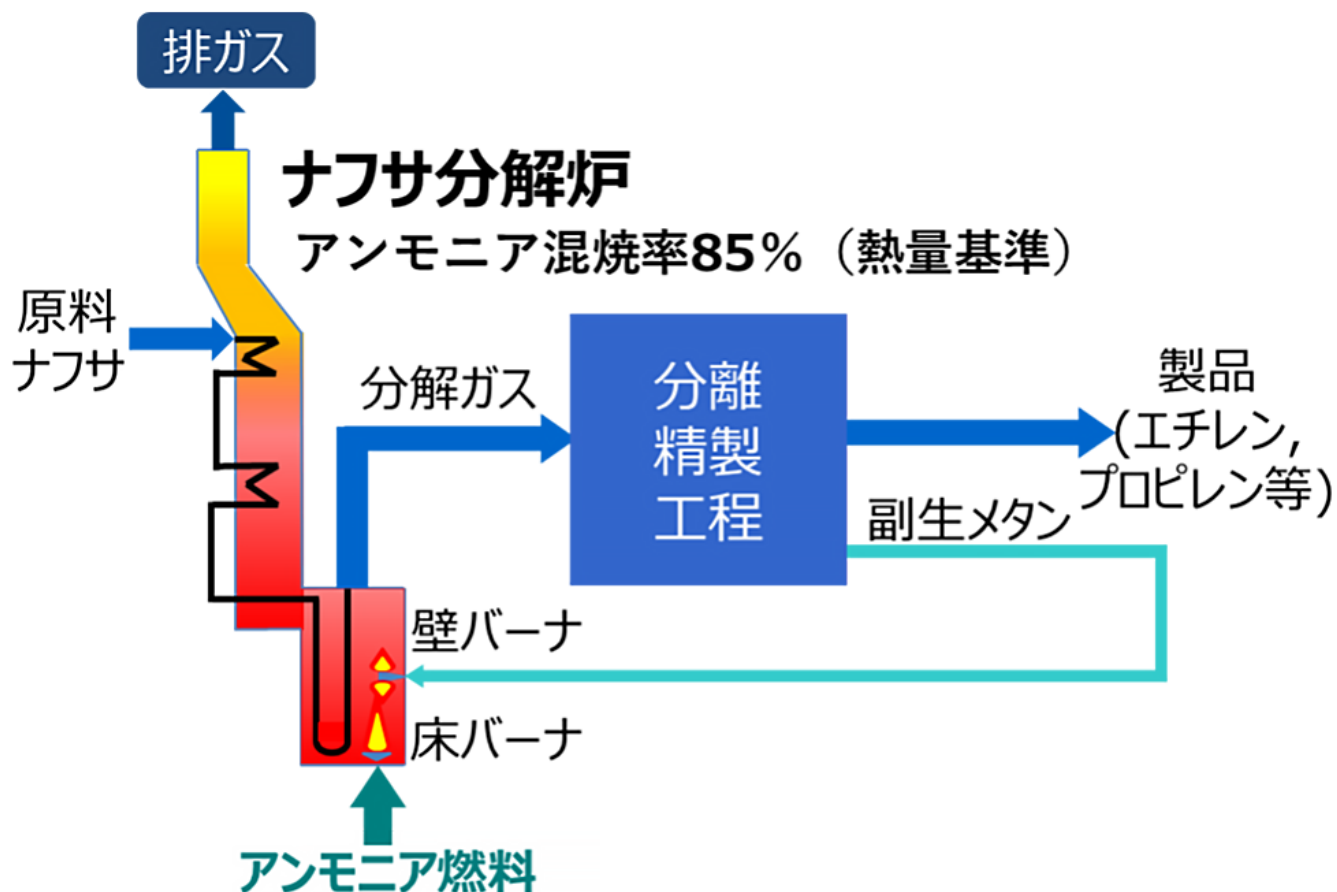
図1 ナフサ分解炉概念図
