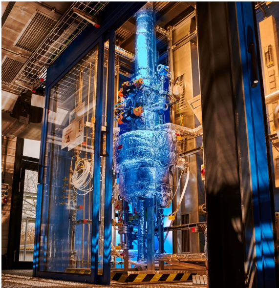
エボニック社 ケミカルリサイクルパイロットプラント（ドイツ）
